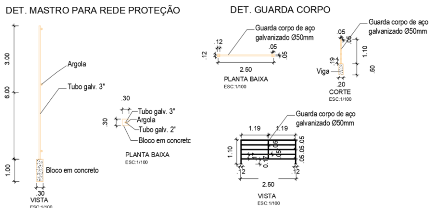
Figura 5 – Detalhes do mastro para rede de proteção e guarda corpo
